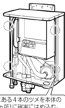
前板の取付けかた
